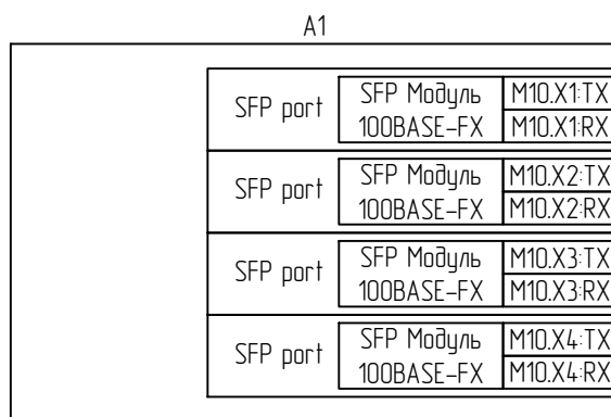
Цели портів зв'язи термінала
